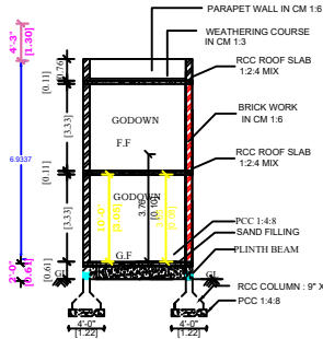
SECTION - AB
