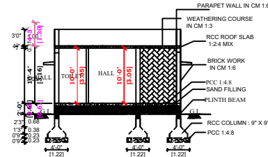
SECTION - AB
