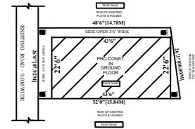
SITE PLAN: SCALE: 1:200
