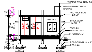
SECTION - AB
