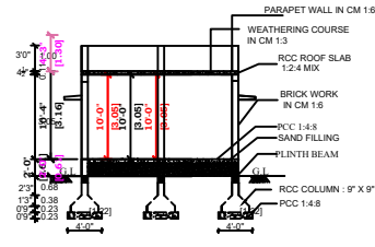
SECTION - AB
