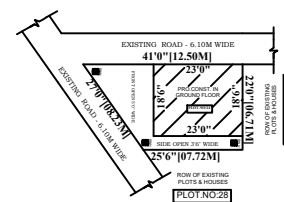
SITE PLAN: SCALE: 1:200
