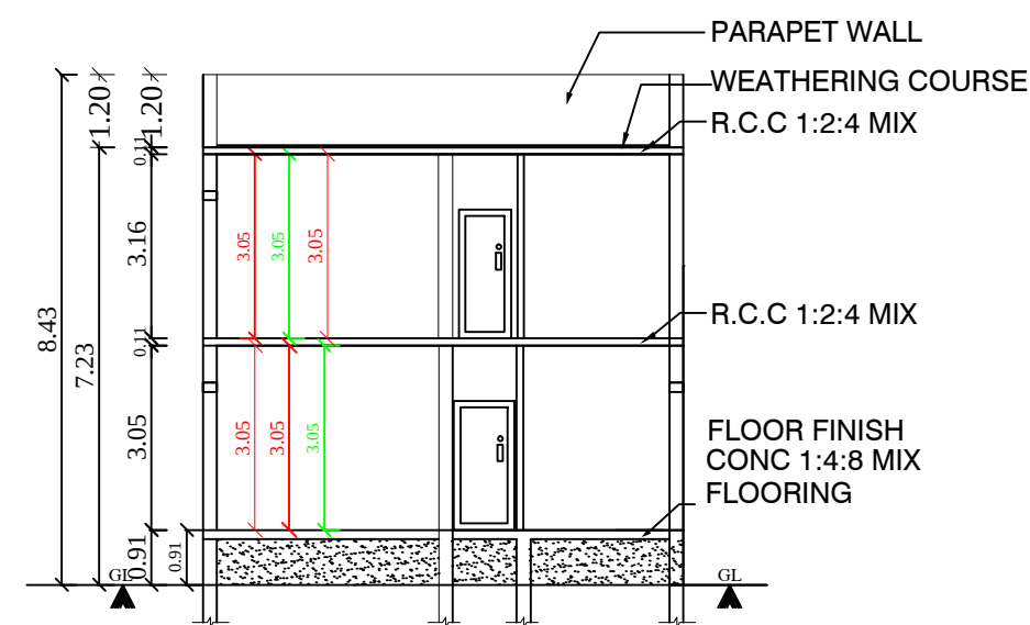
SECTION : "A-A" (SCALE: 1CM : 1M)
