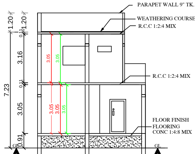
SECTION : "A-A" (SCALE: 1CM : 1M)
