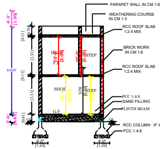
SECTION - AB
