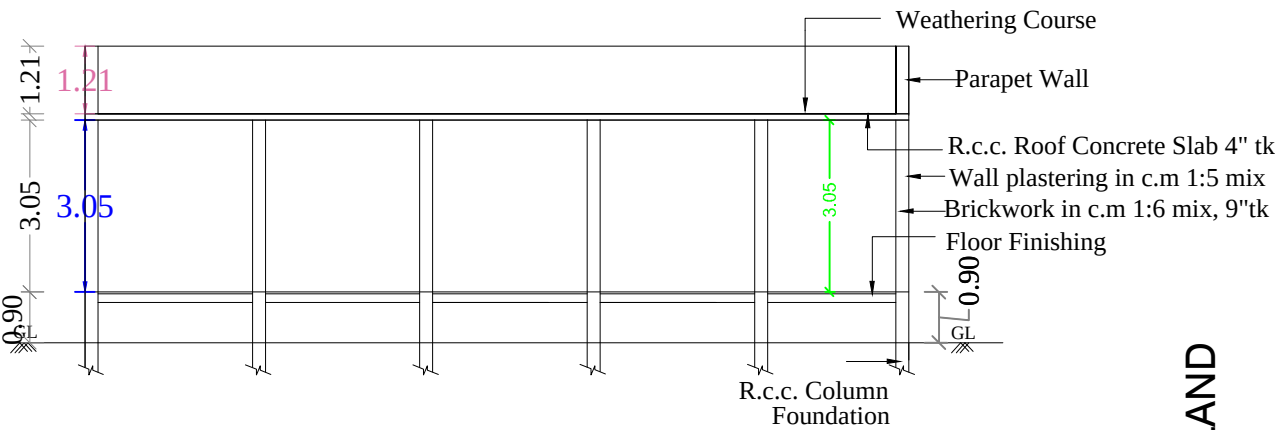
SECTION ON AA SCALE: 1CM: 2M
