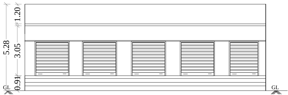
ELEVATION
