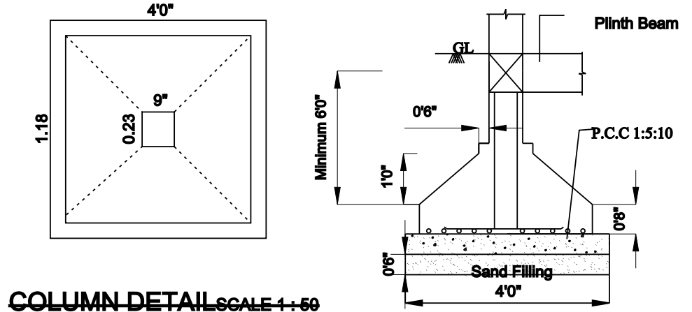
COLUMN-DETAIL SCALE: 1:40
