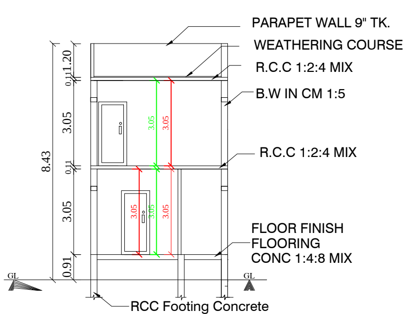
SECTION : "A-A" (SCALE: 1CM : 1M)
