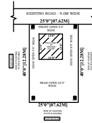
SITE PLAN: SCALE: 1:200
