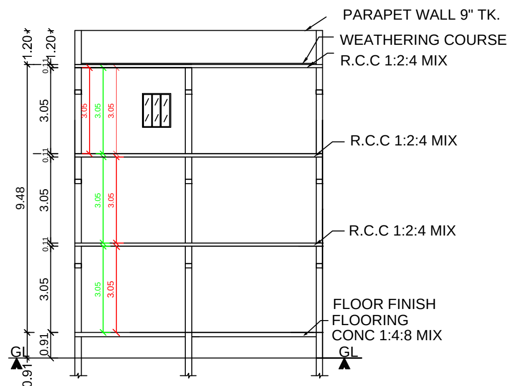
SECTION : "A-A" (SCALE: 1CM : 1M)
