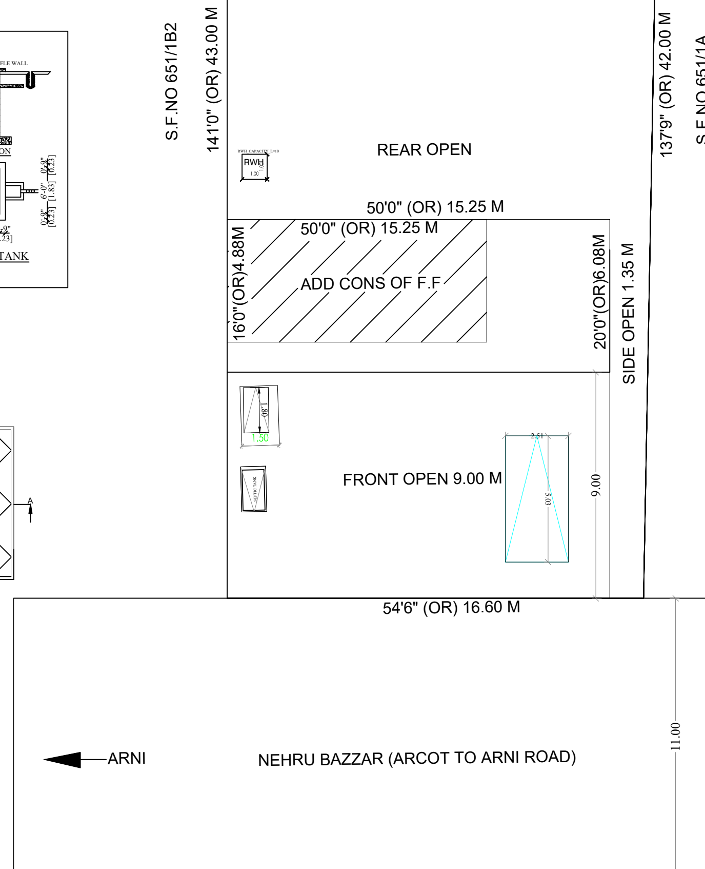
SITE PLAN - SCALE 1:1
