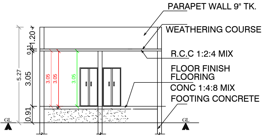
SECTION : "S-J" (SCALE: 1CM : 1M)
