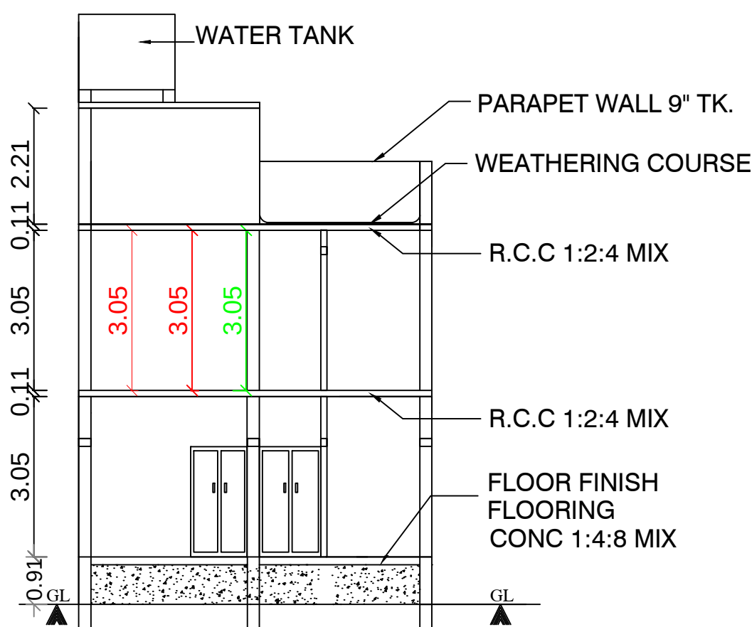
SECTION : "S-J" (SCALE: 1CM : 1M)
