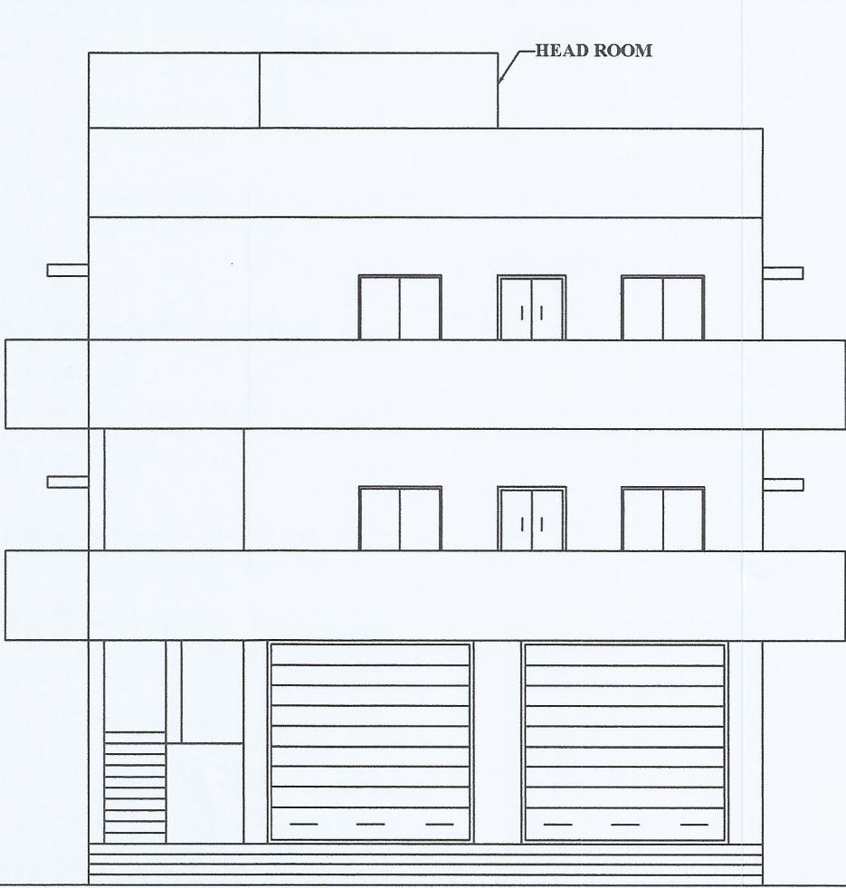
ELEVATION
