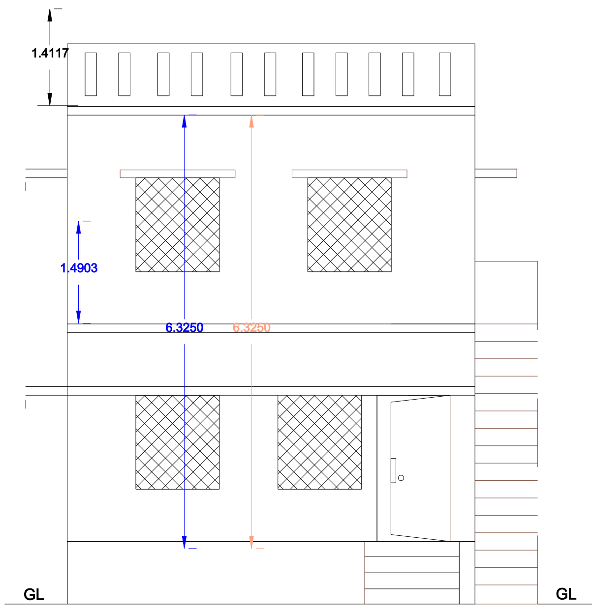
ELEVATION
