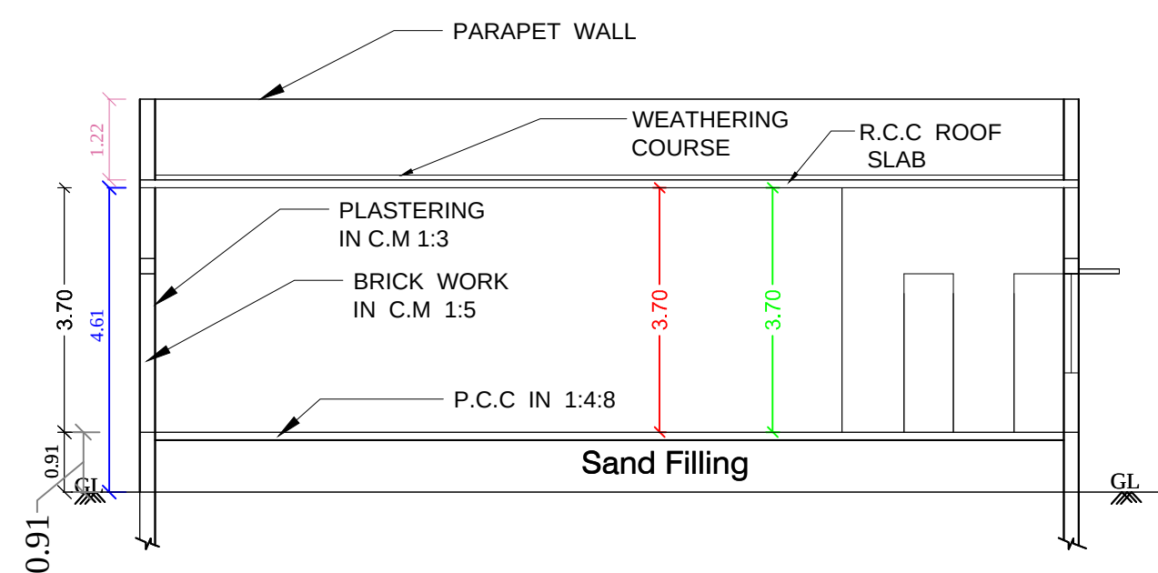
SECTION ON JJ SCALE: 1CM : 1M
