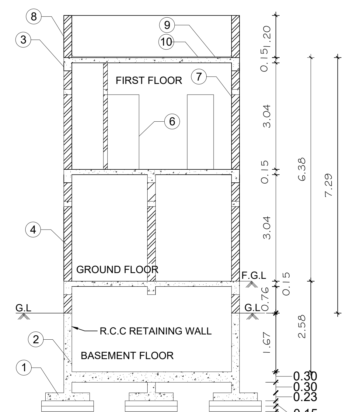
SECTION - AB
