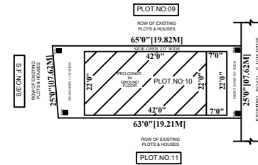
SITE PLAN: SCALE: 1:200
