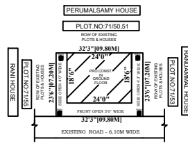
SITE PLAN: SCALE: 1:200
