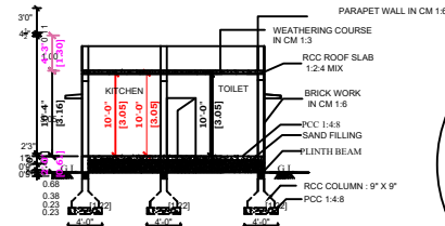
SECTION - AB
