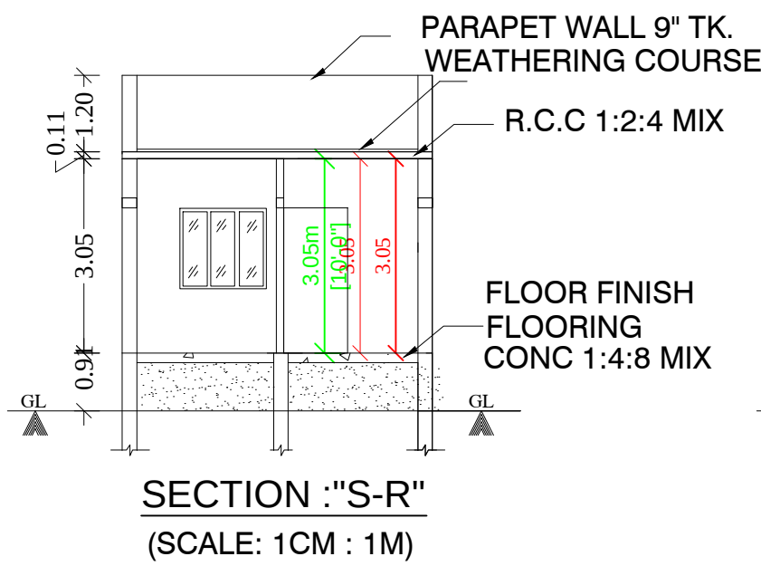
SECTION : "S-R" (SCALE: 1CM : 1M)
