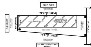
SITE PLAN: SCALE: 1:200
