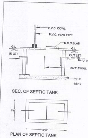
SEPTIC TANK (N.T.S)
