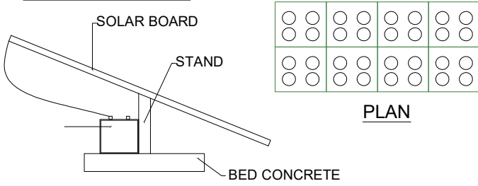
LONGITUDINAL SECTION
