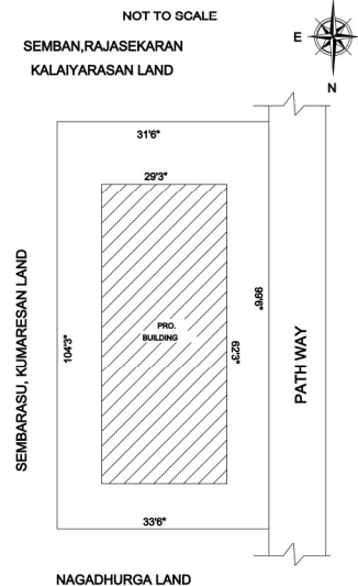
SITE PLAN:-
