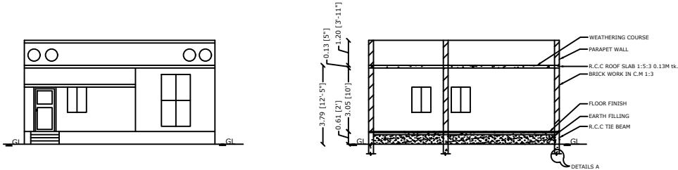
ELEVATION
