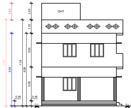
ELEVATION-A
