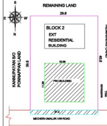
KEY/SITE PLAN:(N.T.S)
