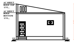
ELEVATION
