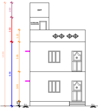
ELEVATION-A
