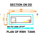
PLAN OF R.W.H. TANK
