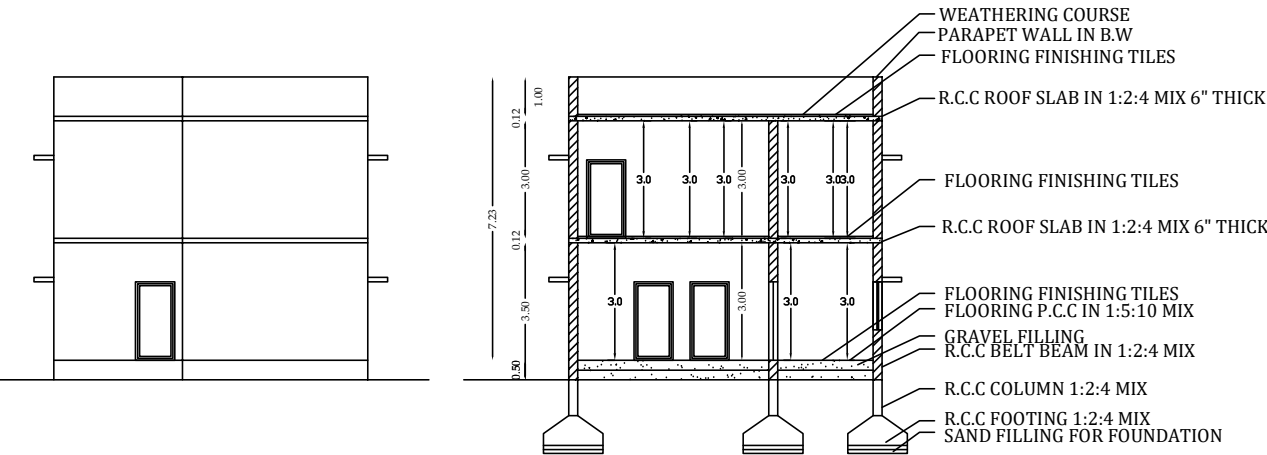
ELEVATION
