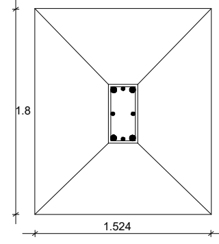
PLAN (N.T.S)
