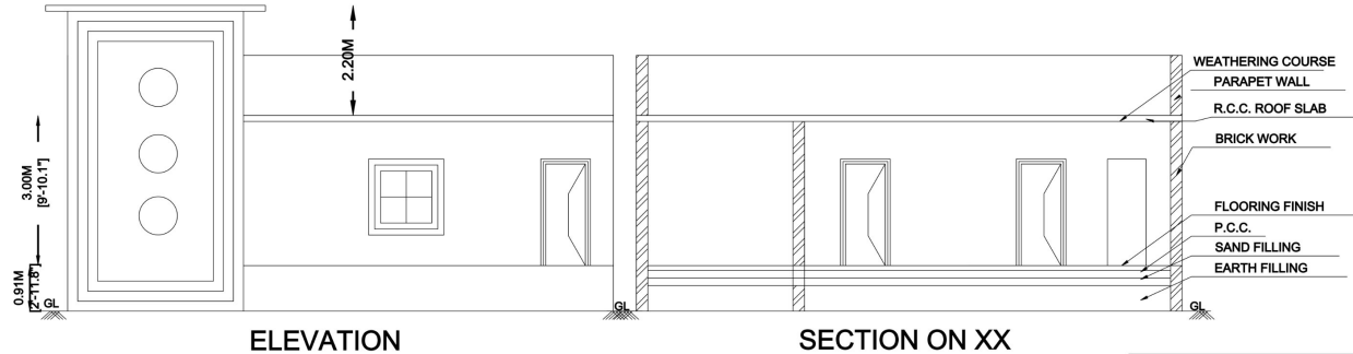
ELEVATION
