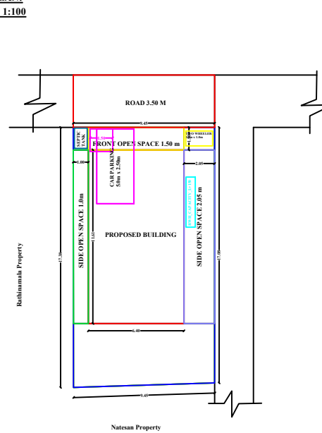
SITE PLAN: SCALE 1:100
