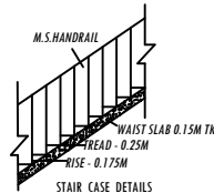
SE DETAILS
