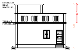
ELEVATION
