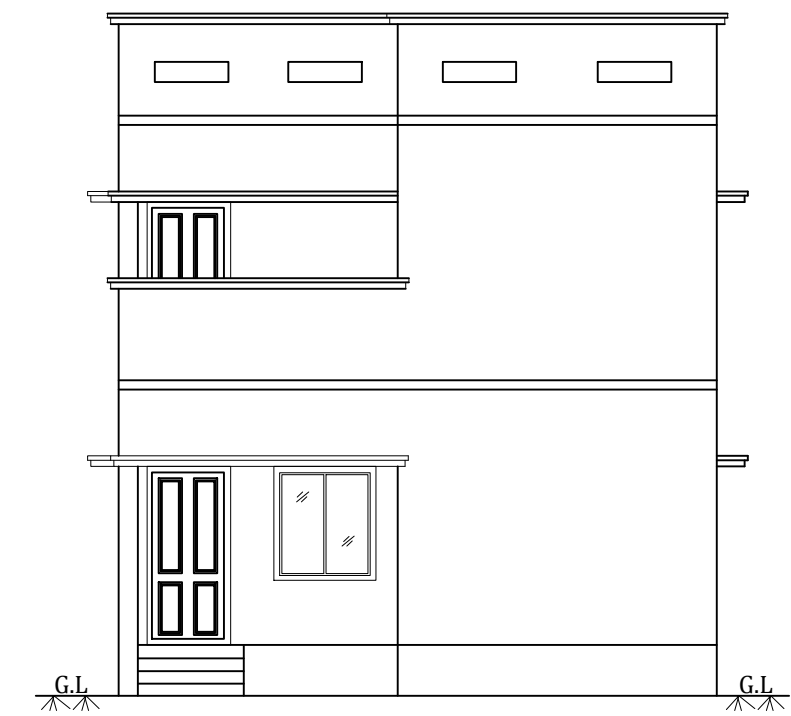
ELEVATION
