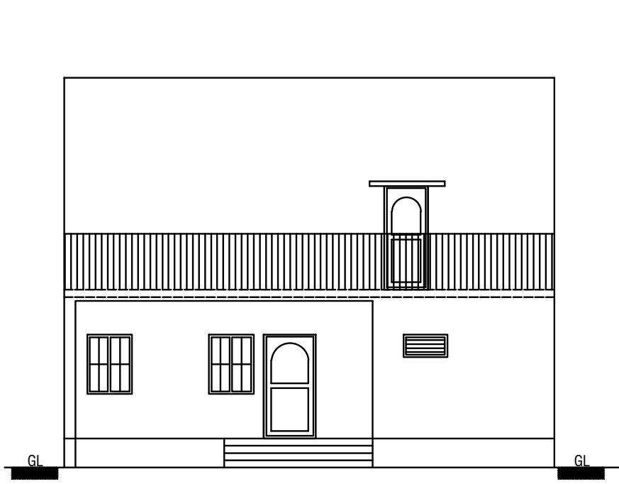
ELEVATION
