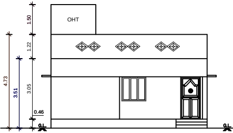
ELEVATION-A
