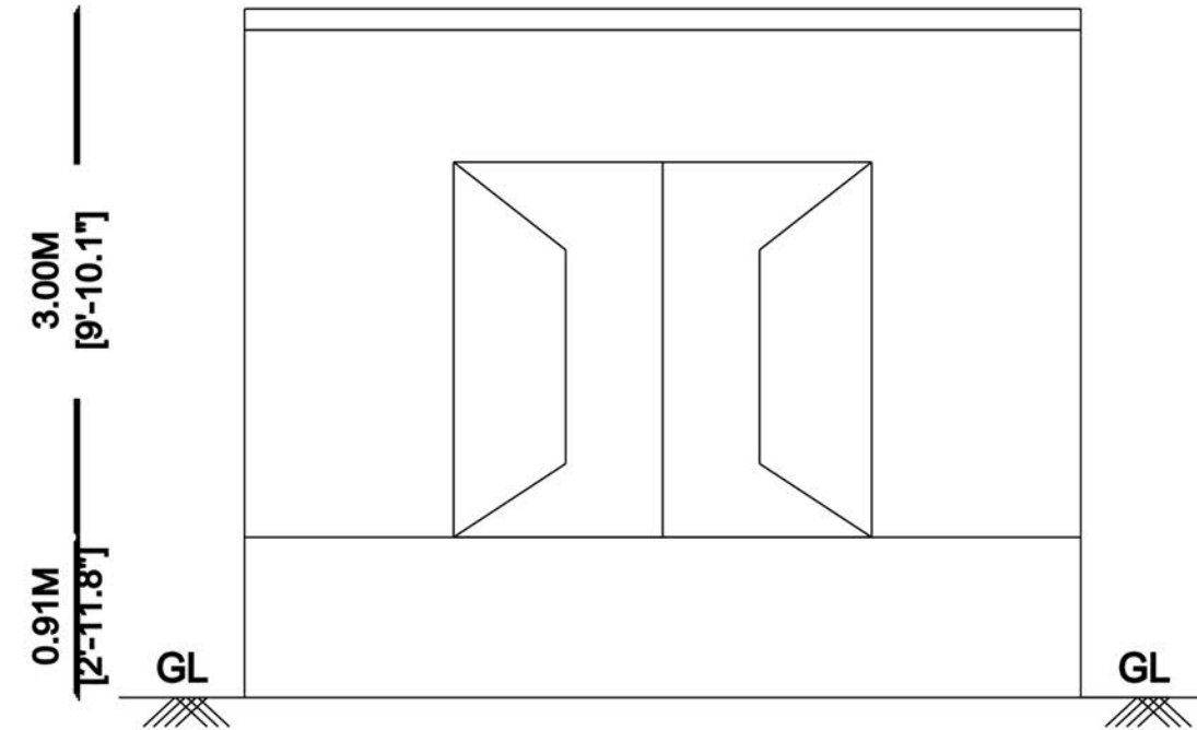
ELEVATION
