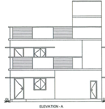
ELEVATION - A
