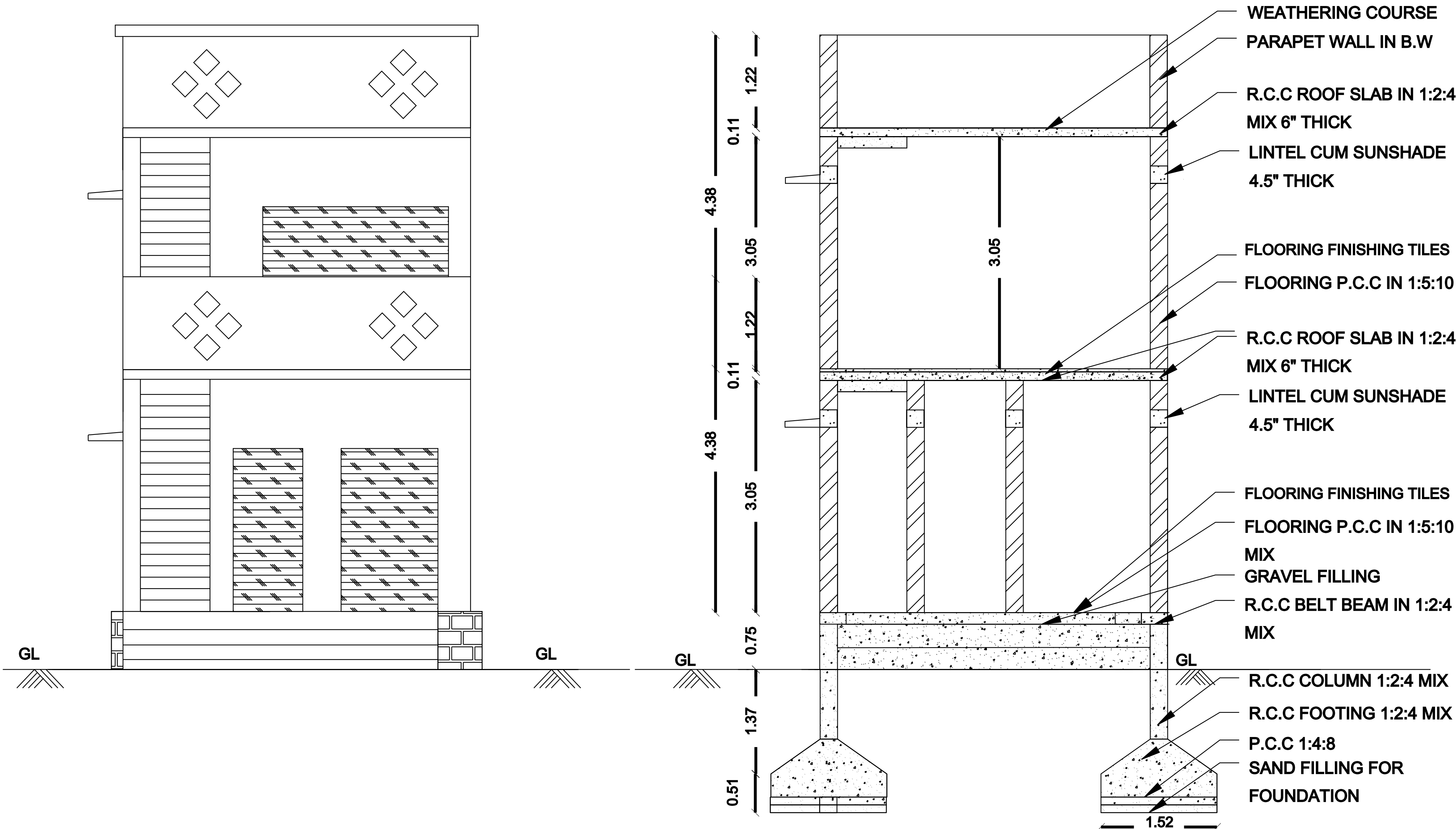
ELEVATION
