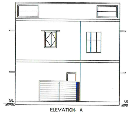
ELEVATION - A
