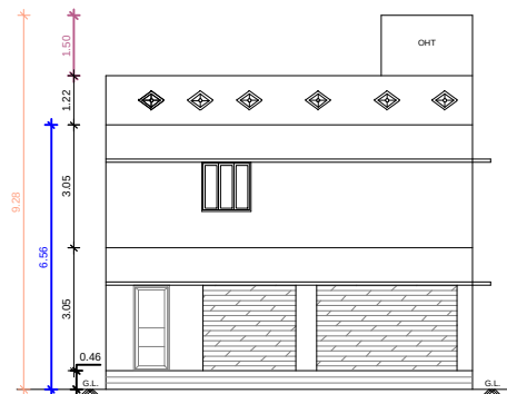
ELEVATION-A
