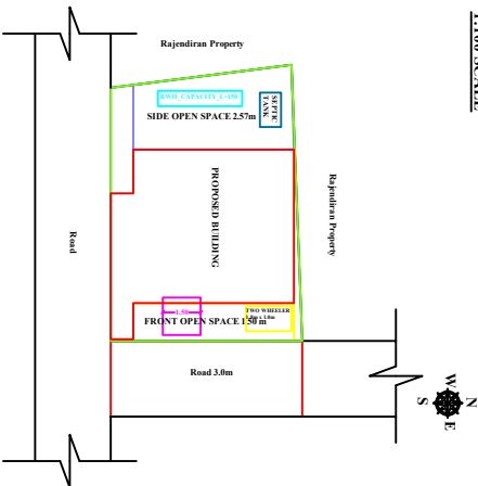
SITE PLAN 1:100 SCALE
