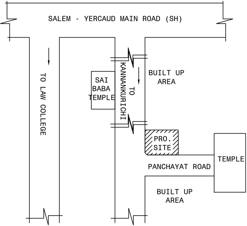
SITE PLAN (1:150)
