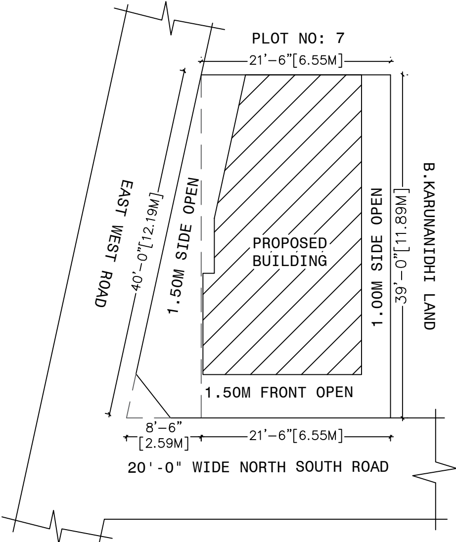
SITE PLAN (1:150)
