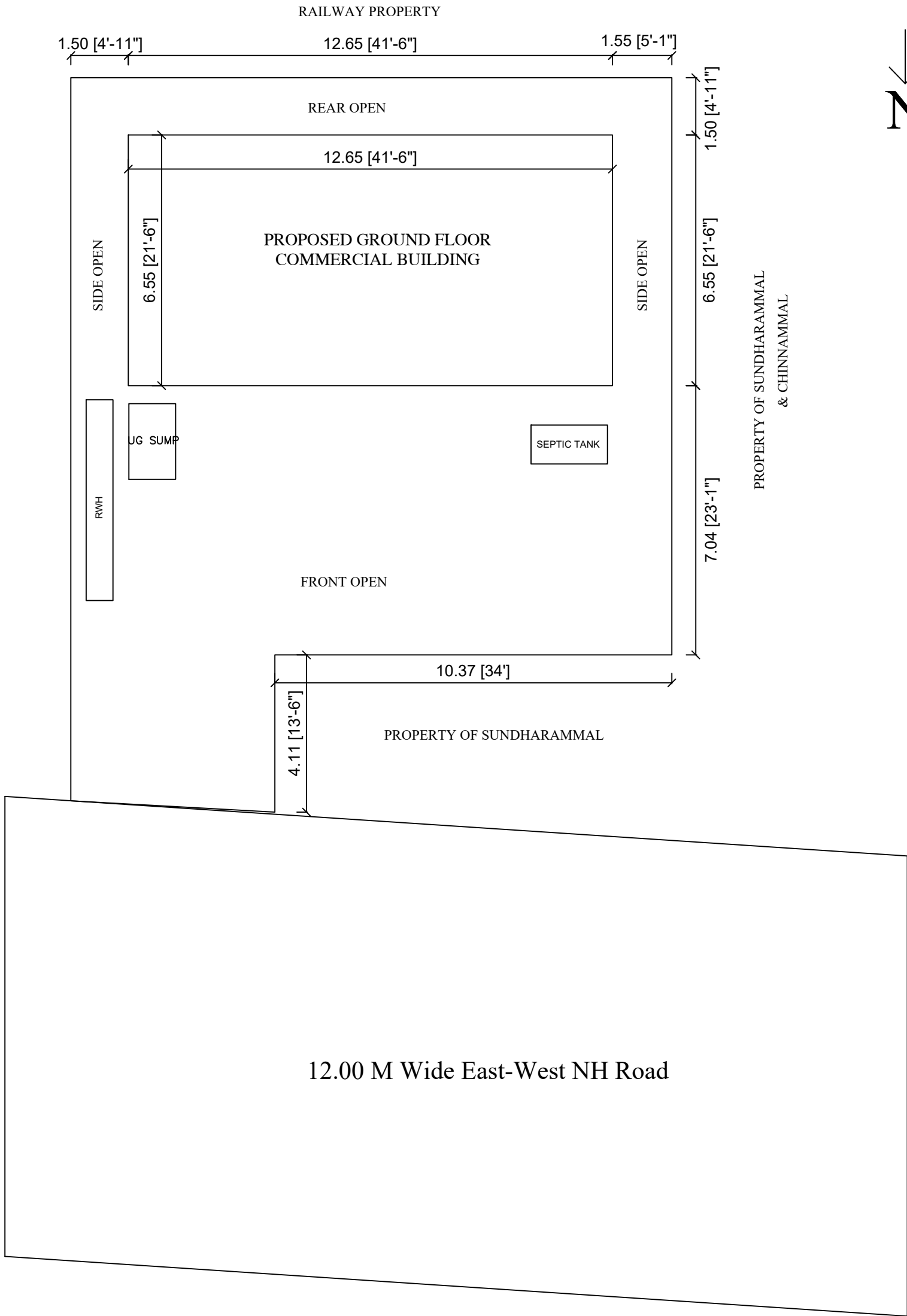
SITE PLAN 1:100
