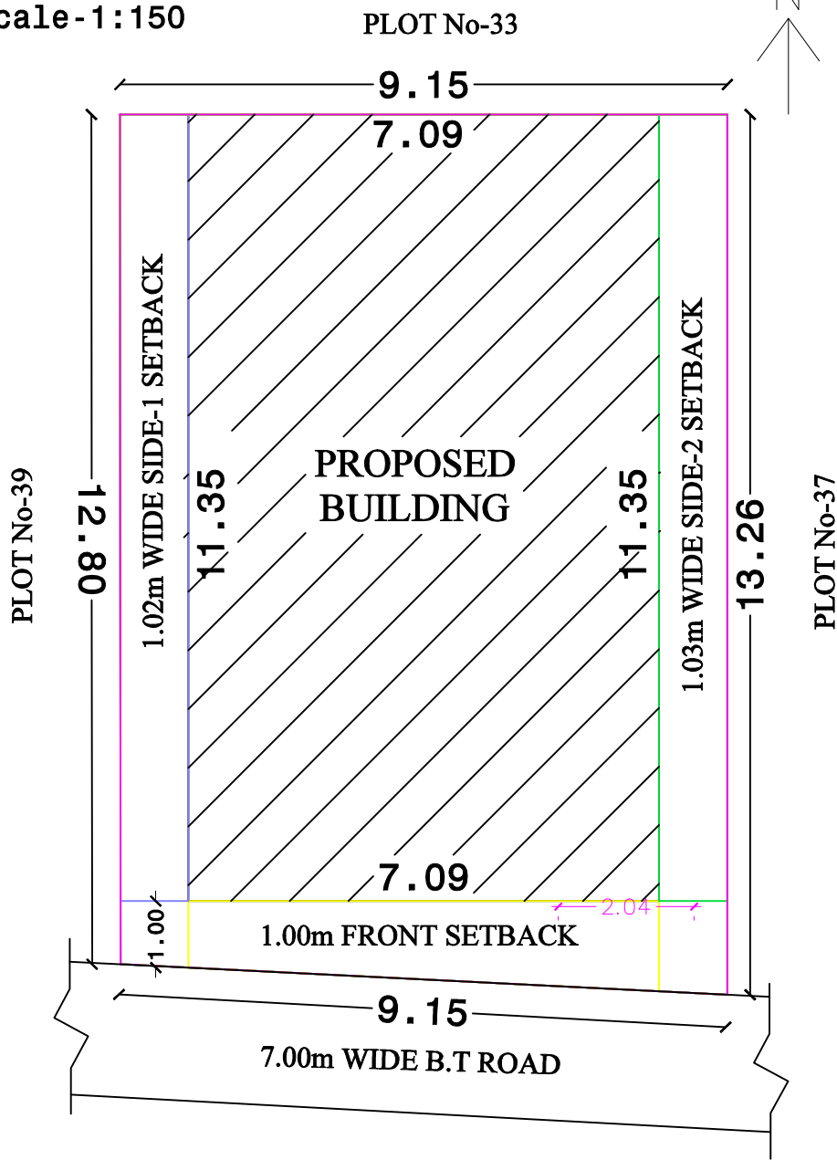
SITE PLAN: Scale-1:150
